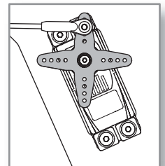
Heckservoarm in neutraler Position (betrachtet von der rechten Seite)
