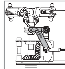
Heck-Pitchschieber in neutraler Position (betrachtet von Unterseite)
