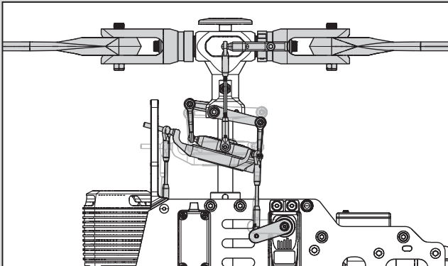
Nicken nach hinten (von links betrachtet)
