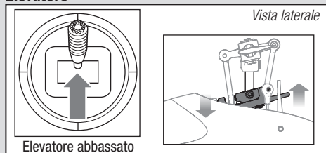
Elevatore abbassato
