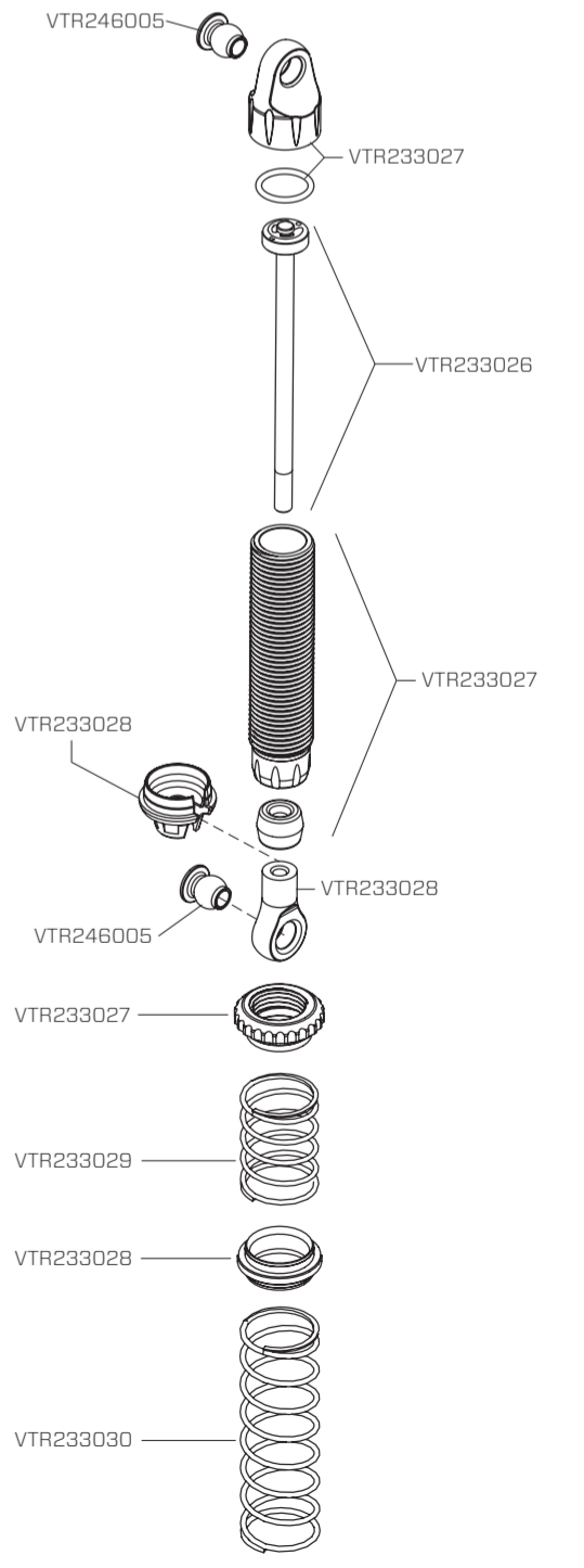
SHOCK ASSEMBLY STÖßDÄMPFER MONTAGE ASSEMBLAGE D'UN AMORTISSEUR GRUPPO AMMORTIZZATORE
