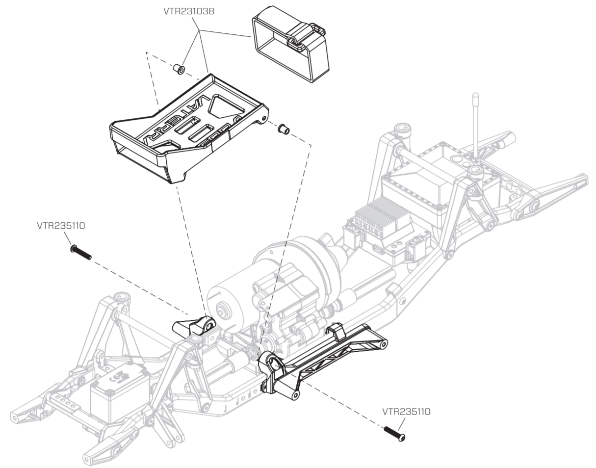
BATTERY TRAY ASSEMBLY MONTAGE DES AKKUHALTERS ASSEMBLAGE DU SUPPORT DE BATTERIE GRUPPO SUPPORTO BATTERIA
