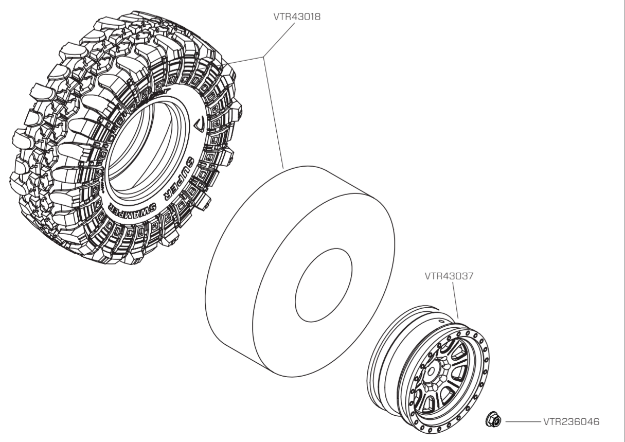
WHEEL AND TIRE ASSEMBLY MONTAGE FELGEN UND REIFEN MONTAGE DU PNEU SUR LA JANTE ASSEMBLAGGIO CERCHI E GOMME
